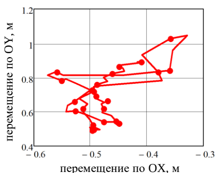
Рисунок 5 – Годограф ЦМ 4-го звена (туловище). Вес 100 кг
