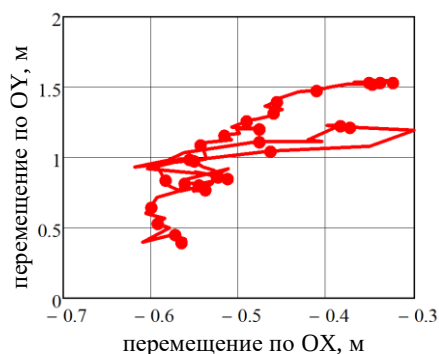
Рисунок 4 – Годограф ЦМ 6-го звена (предплечье). Вес 140 кг
