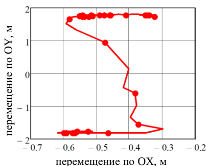
Рисунок 8 – Годограф грифа штанги. Вес 140 кг
