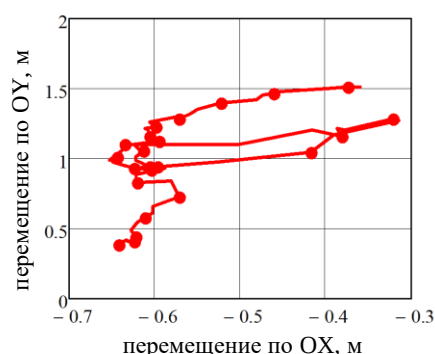
Рисунок 6 – Годограф ЦМ 6-го звена (предплечье). Вес 100 кг
