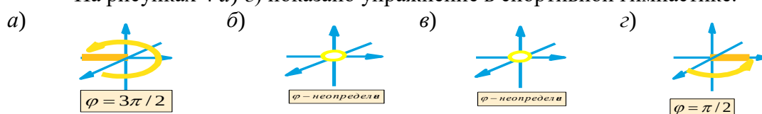
Рисунок 3 – Неопределенность угла \varphi в сферической системе координат
