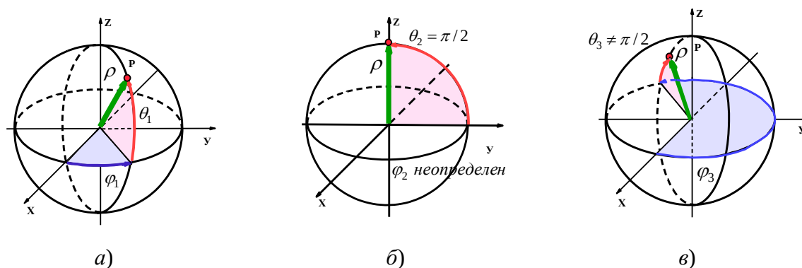
Рисунок 3 – Неопределенность угла \varphi в сферической системе координат
